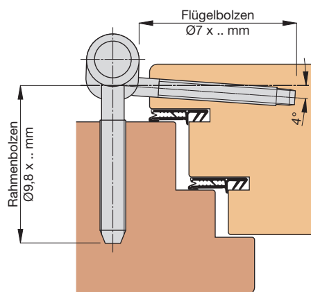
Mit Dichtung im Überschlag - TOP320...S2, S3, S9
